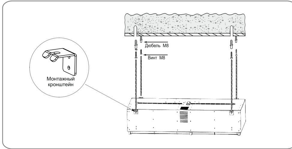
МЕЖЦЕНТРОВЫЕ РАССТОЯНИЯ ОТВЕРСТИЙ КРЕПЛЕНИЯ ВОЗДУШНЫХ ЗАВЕС
