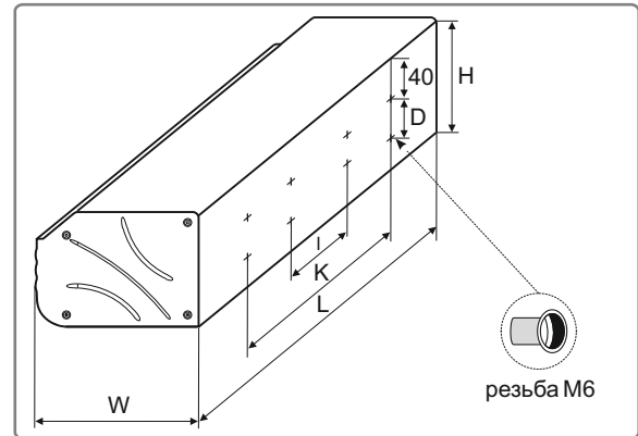
МЕЖЦЕНТРОВЫЕ РАССТОЯНИЯ ОТВЕРСТИЙ КРЕПЛЕНИЯ ВОЗДУШНЫХ ЗАВЕС
