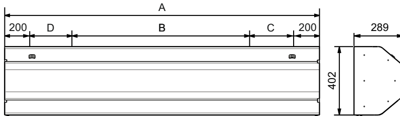
МЕЖЦЕНТРОВЫЕ РАССТОЯНИЯ ОТВЕРСТИЙ КРЕПЛЕНИЯ ВОЗДУШНЫХ ЗАВЕС
